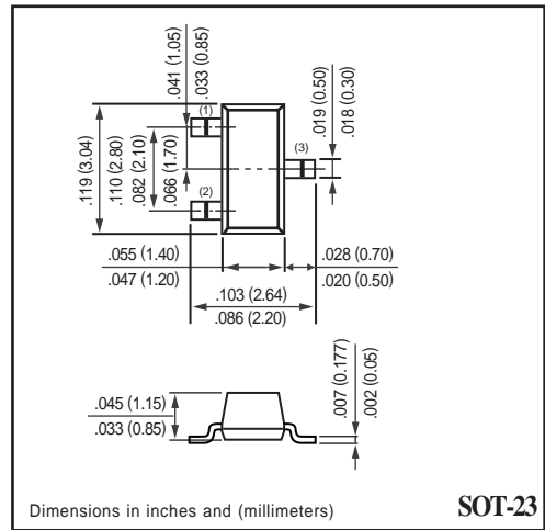
SOT-23
